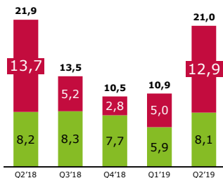
■ OZE (TWh)
